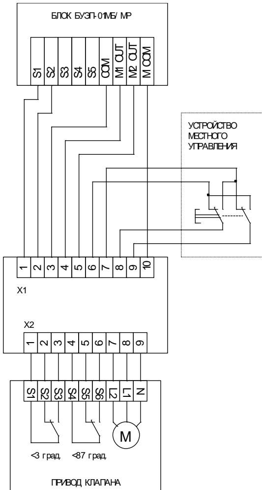
Однофазно реверсивный привод с местным управлением
