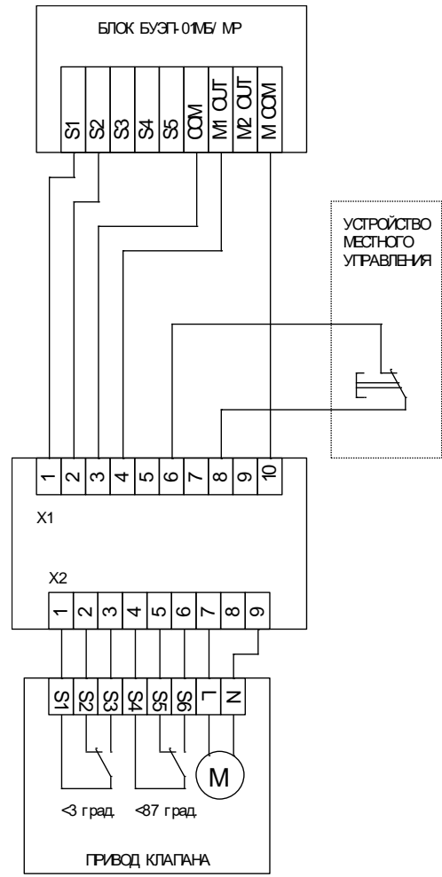
Привод с возвратной пружиной с местным управлением
