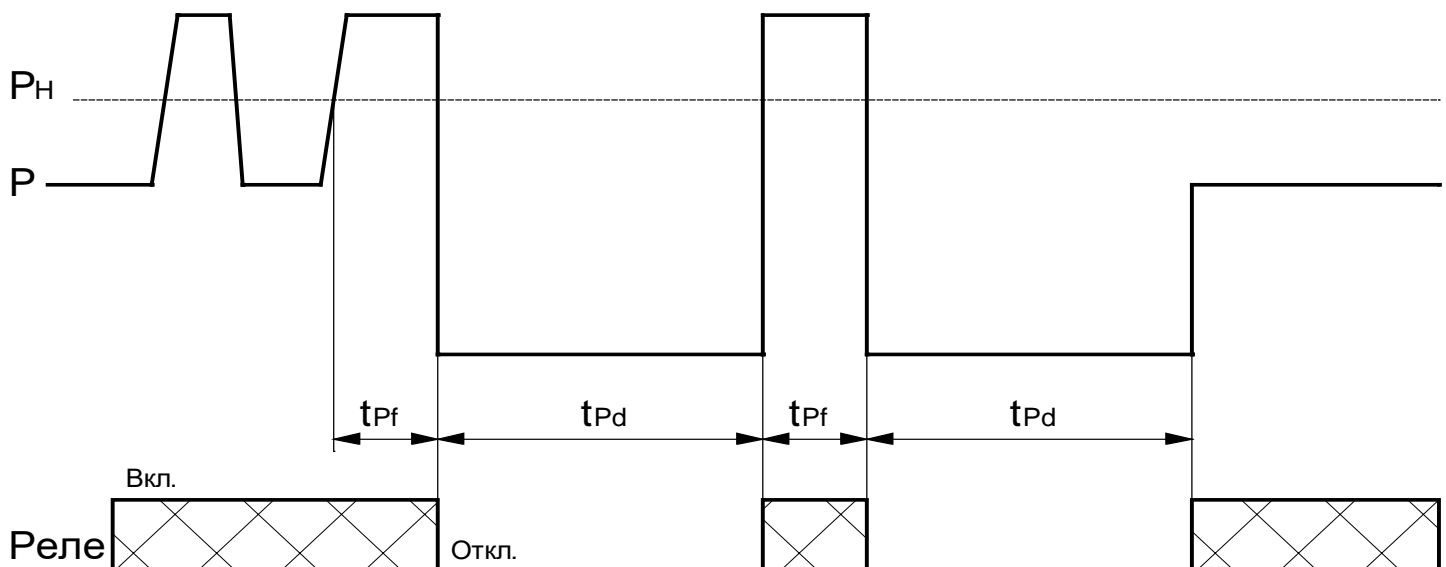
Рисунок 4 – Диаграмма работы устройства в режиме ограничения мощности
