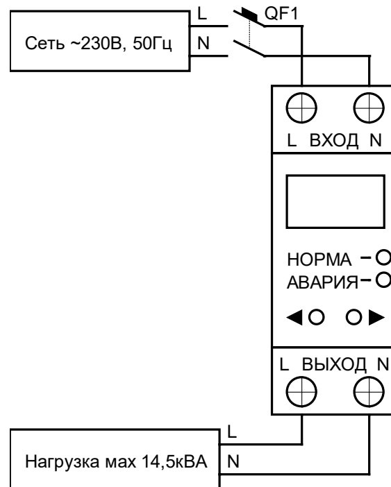
Рисунок 2 – Схема подключения устройства
