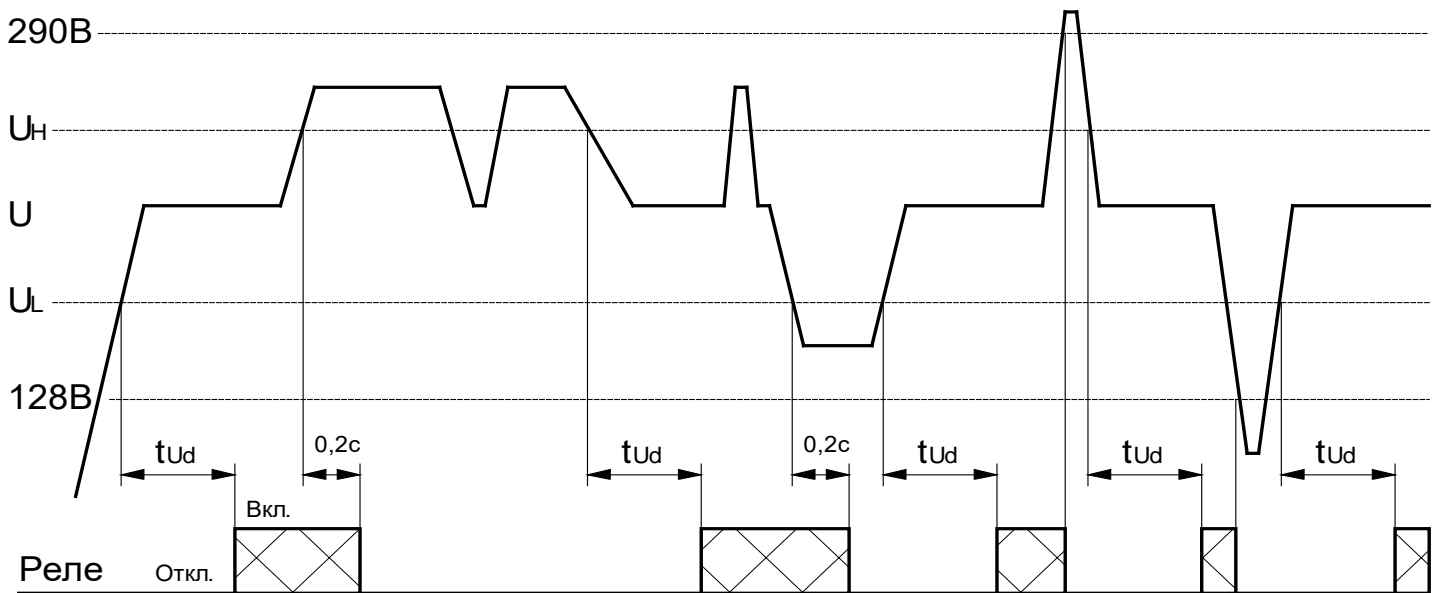
Рисунок 3 – Диаграмма работы устройства в режиме контроля напряжения
