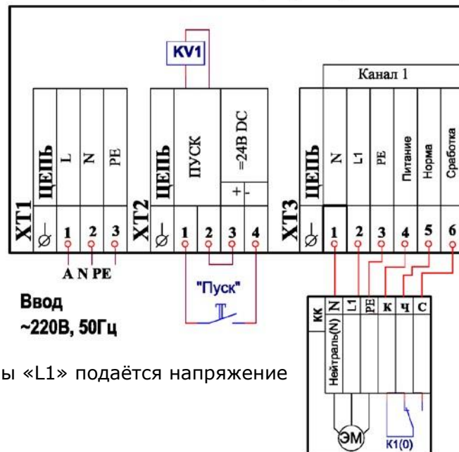
Пример подключения на канал №1 клапана с электромагнитным приводом "Belimo" ~220В:
