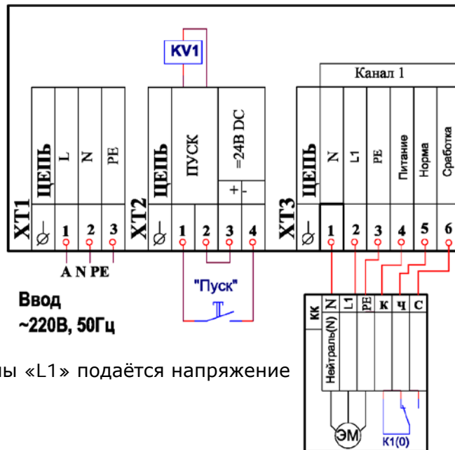
Пример подключения на канал №1 клапана с электромагнитным приводом "Velimo" ~220В:
